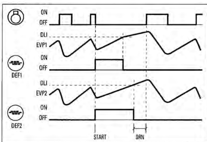
Рисунок 2. Функционирование оттайки
